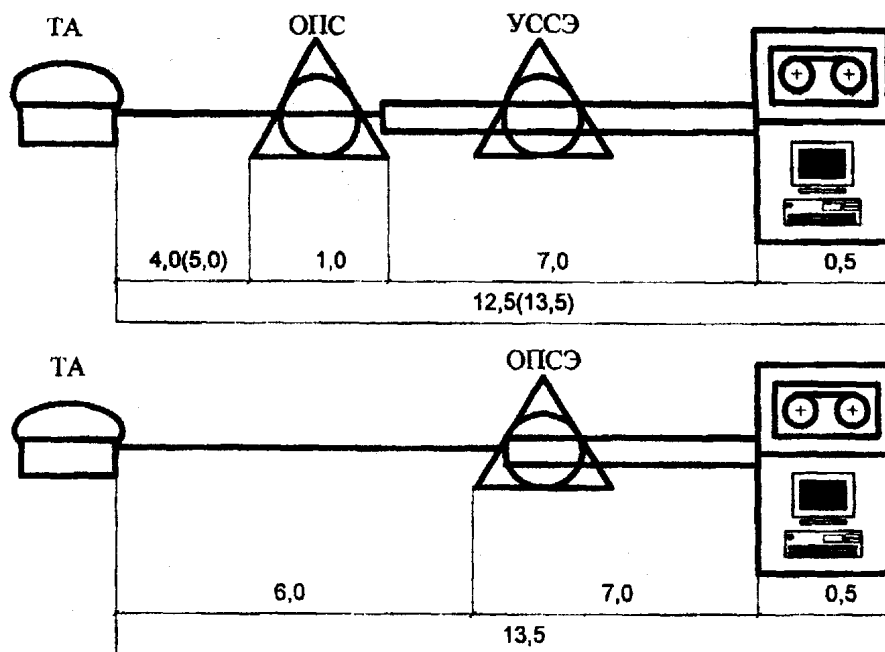
Рисунок Б.6 - Распределение норм затухания для абонентов междугородной связи ГТС
