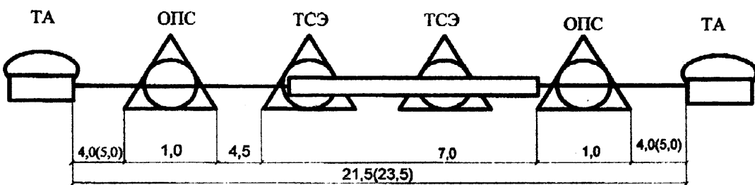
Рисунок Б.5 - Распределение норм затухания на районированной ГТС с узлами исходящего и входящего сообщения, лист 1
