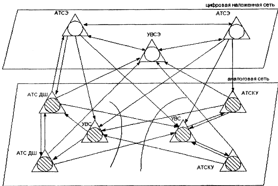
Рисунок 6.2 - Структура аналого-цифровой сети с узлами входящих сообщений
