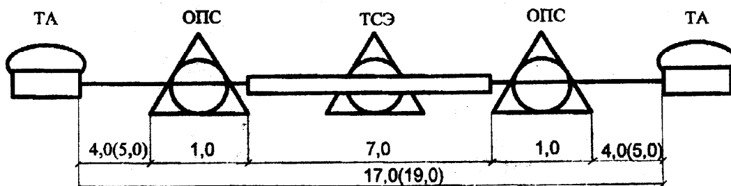
Рисунок Б.4 - Распределение норм затухания на районированной ГТС с узлами входящего сообщения
