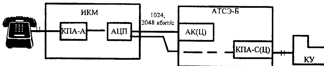
Рис. 6.5. Реализация на АТСЭ-Б цифрового абонентского комплекта для подключения прямого абонента
