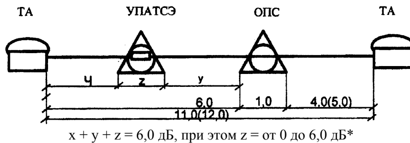
Рисунок Б.1 - Распределение норм затухания на нерайонированной сети, лист 1
